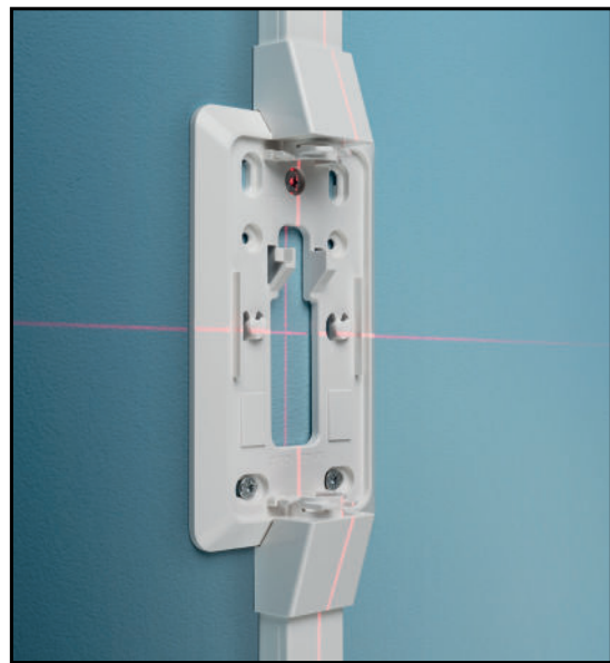
De kabelinvoer P 25 wordt op de montageplaat gemonteerd, vervolgens wordt de kabel ingevoerd.
